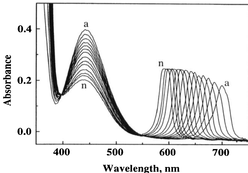
FIGURE 5 Change of cholesteric pitch of eutectic mixture of 5b, at different time intervals after irradiation at 60 °C for 5 min. a) 0 min, b) 5 min, c) 10 min, d) 15 min, e) 20 min, f) 25 min, g) 30 min, h) 40 min, i) 50 min, j) 60 min, k) 80 min, l) 100 min, m) 120 min, n) 200 min
